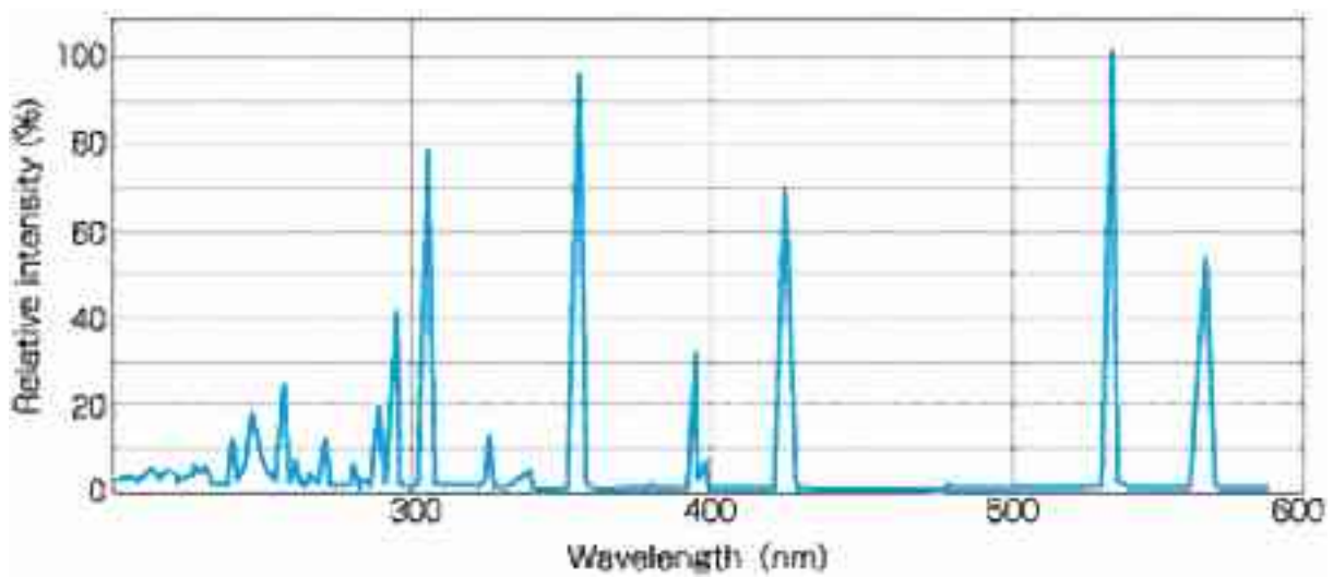
2. kép A 300 wattos higanygőzlámpa emissziós színe
